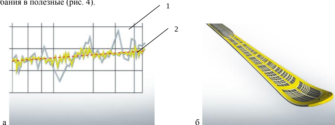
Рис. 4. Амплитудно-частотные характеристики колебаний лыжи (а):
