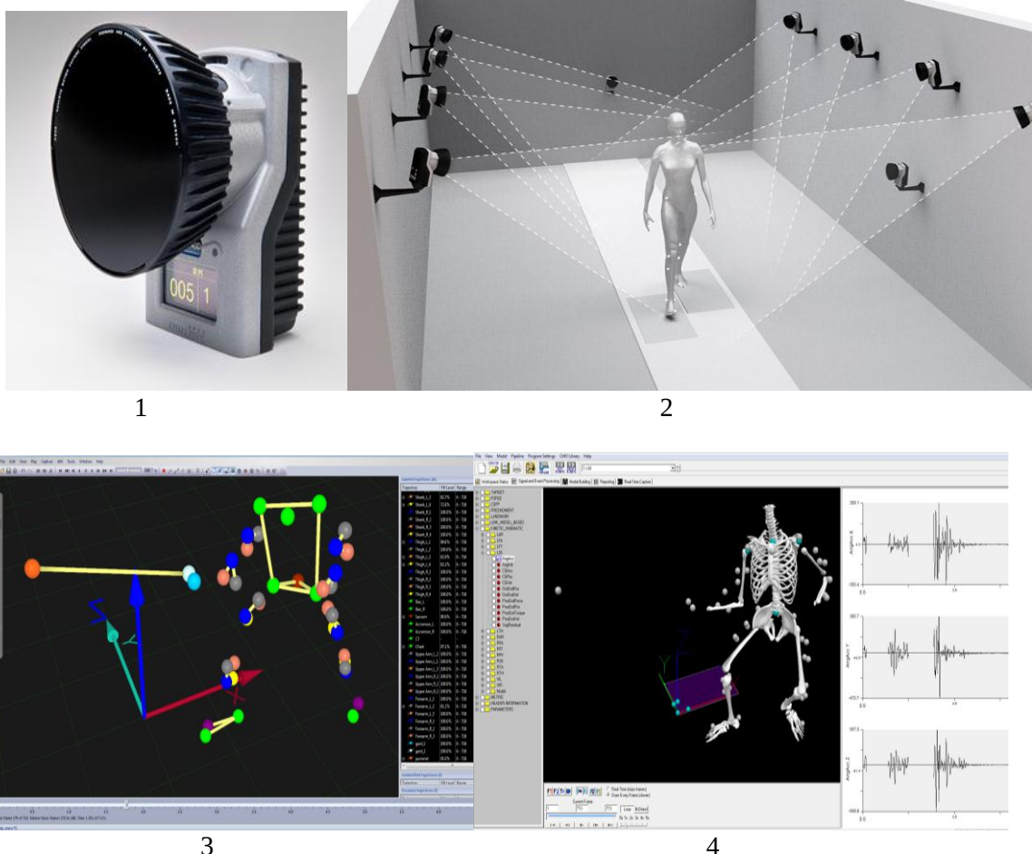
Рис. 6. Оптико-электронная система регистрации и анализа движений тела спортсмена «Qualisys»: 1 – камера «Oqus 7+»; 2 – пример расположения камер системы «Qualisys» при регистрации биомеханических показателей техники двигательных действий спортсмена; 3 – визуализация трехмерной биокинематической модели тела спортсмена и получение количественных показателей техники его движения в программном обеспечении «Qualisys Track Manager»; 4 – «Visual 3D» [9]
